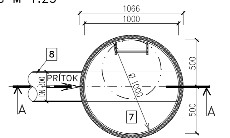
PÔDORYS M 1:25
