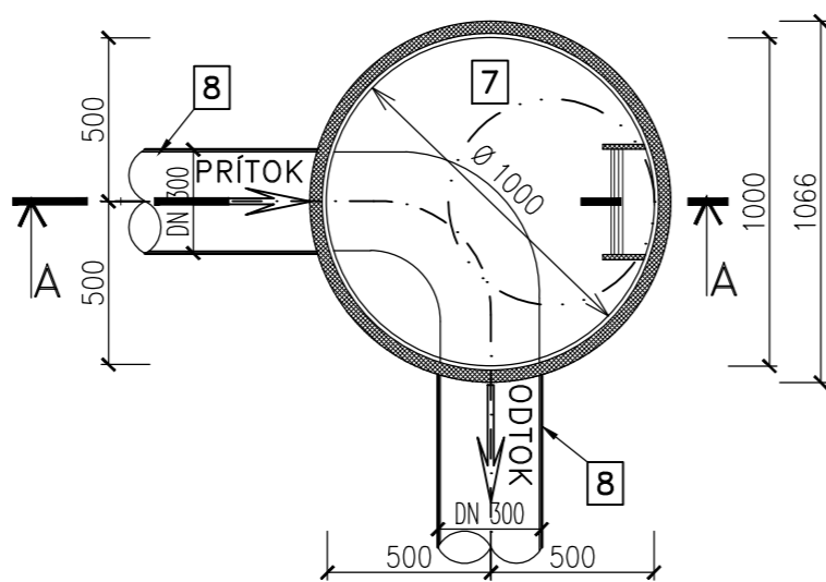
PÔDORYS M 1:25
