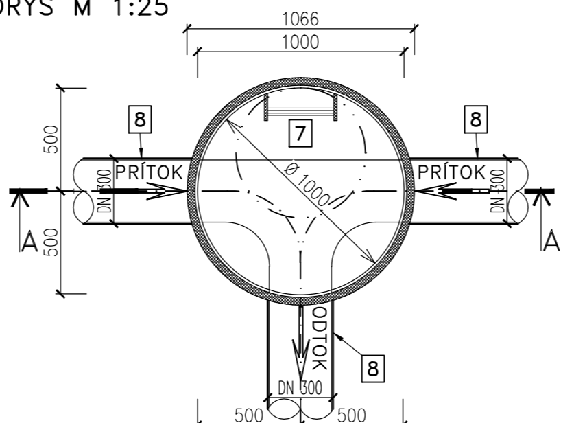
PÔDORYS M 1:25
