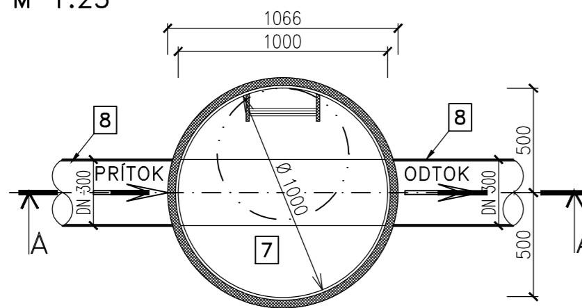
PÔDORYS M 1:25
